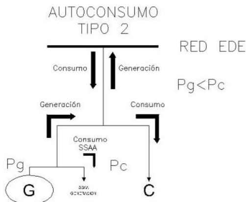
Figura 2. Autoconsumo tipo 2
