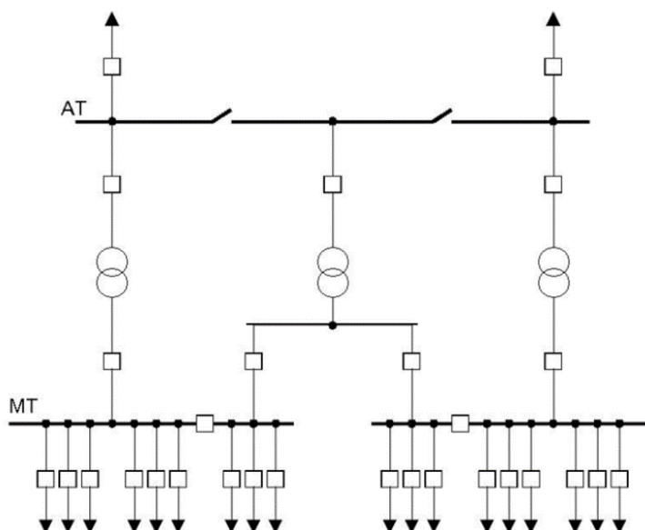
Figura 8. Esquema especial SB
