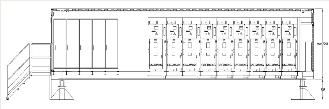
Container GSCM770/2. Alzado.
