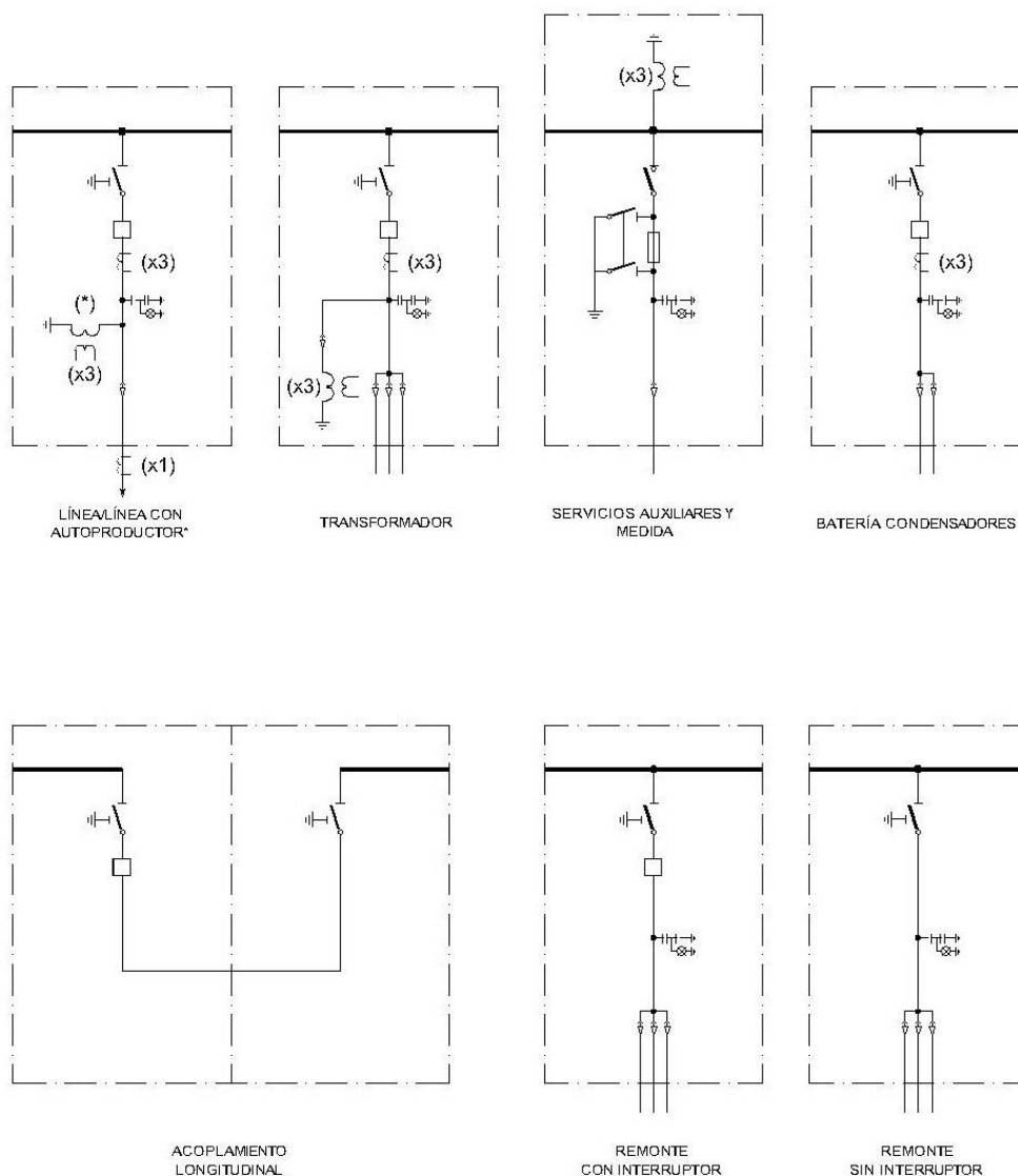
Figura 29. CELDAS MT SIMPLE BARRA
