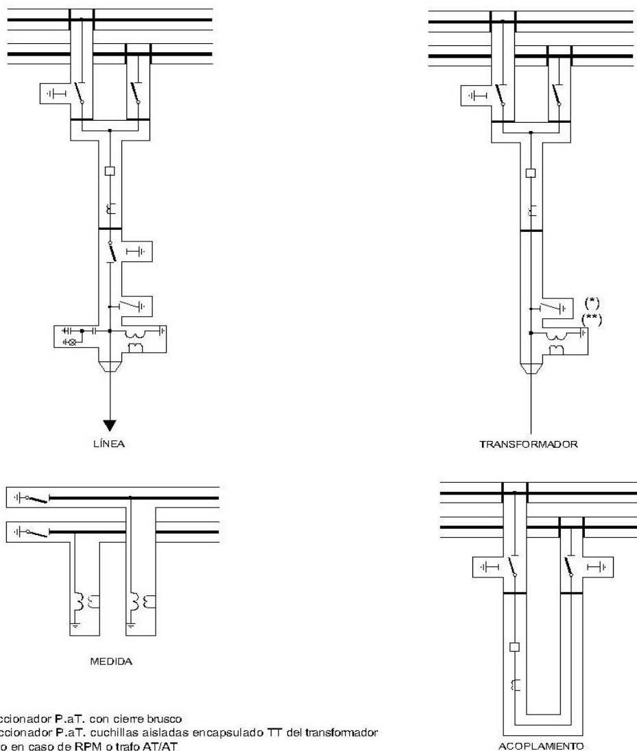
Figura 15. EQUIPO BLINDADO GIS DB (132-110-66 kV)
