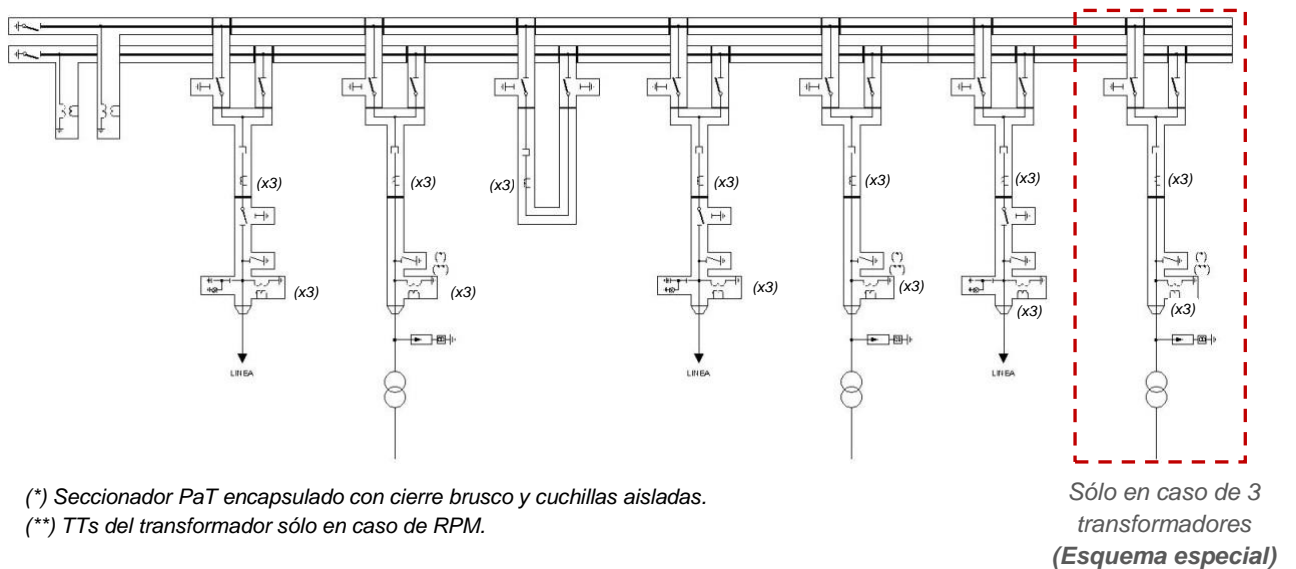
Figura 23. Esquema Unifilar GIS estándar y especial DB
