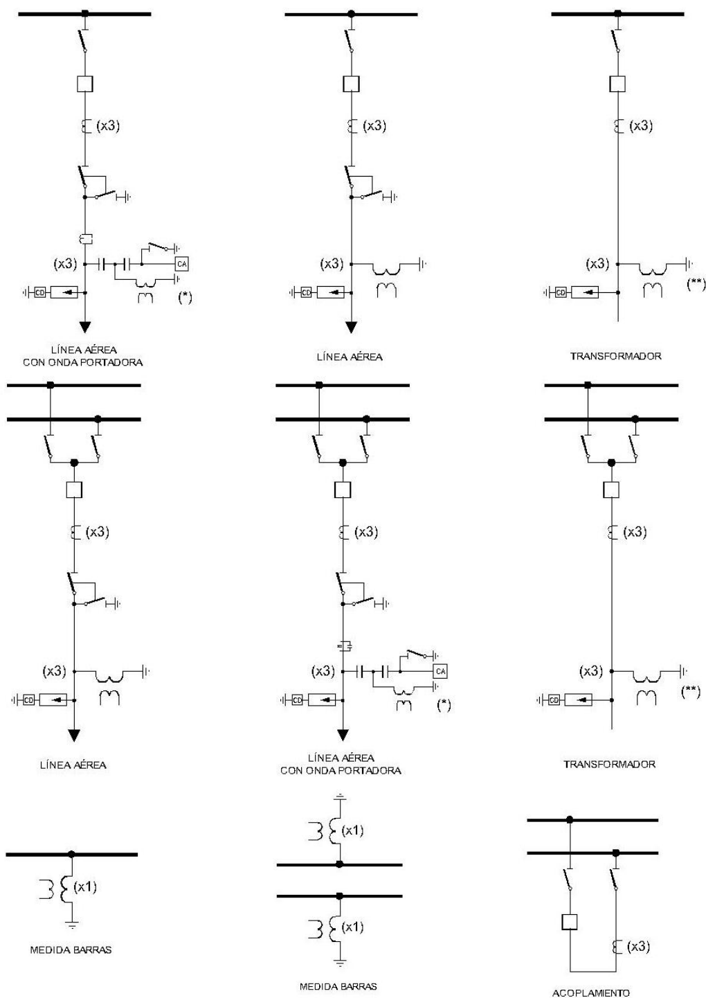
Figura 14. ESQUEMA POSICIONES CONVENCIONALES AT
