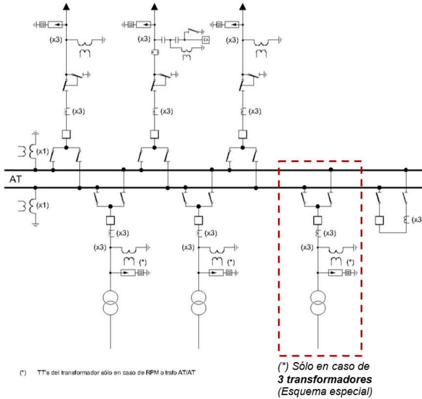
Figura 18. Esquema Unifilar convencional estándar y especial DB
