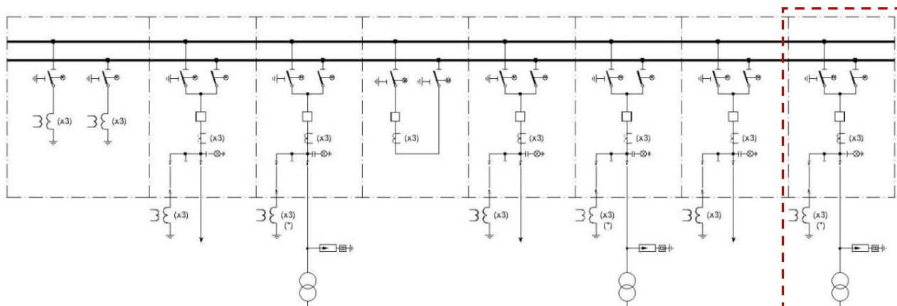
Caso de 3 transformadores (Esquema especial)
