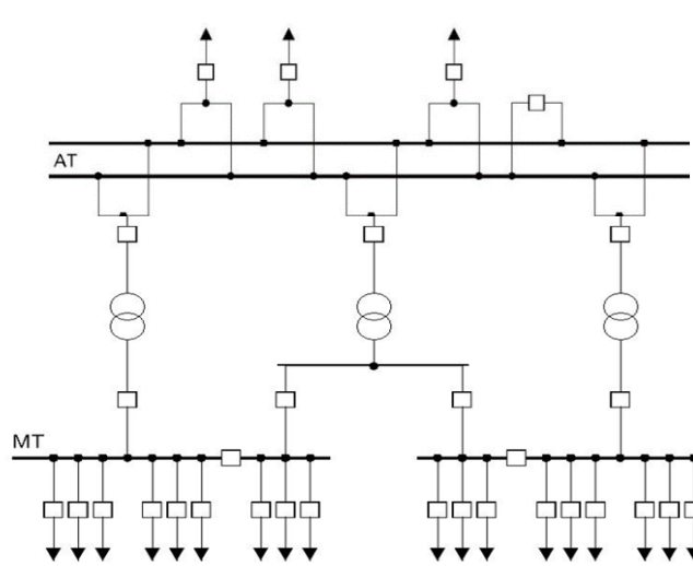
Figura 10. Esquema especial DB (SSEE Nodal)
