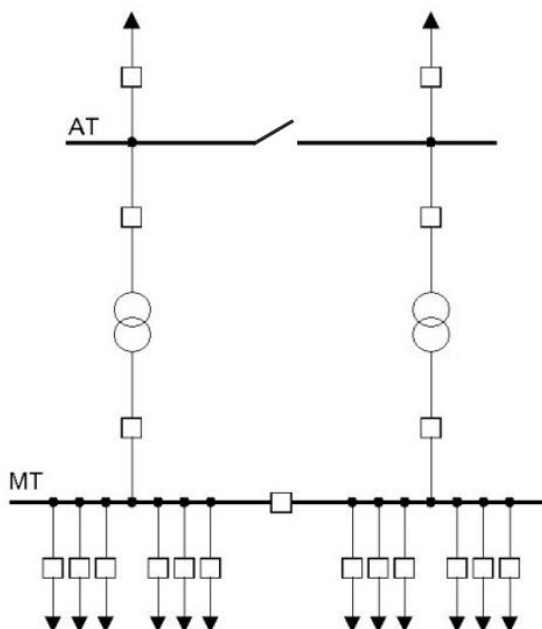
Figura 7. Esquema estándar SB
