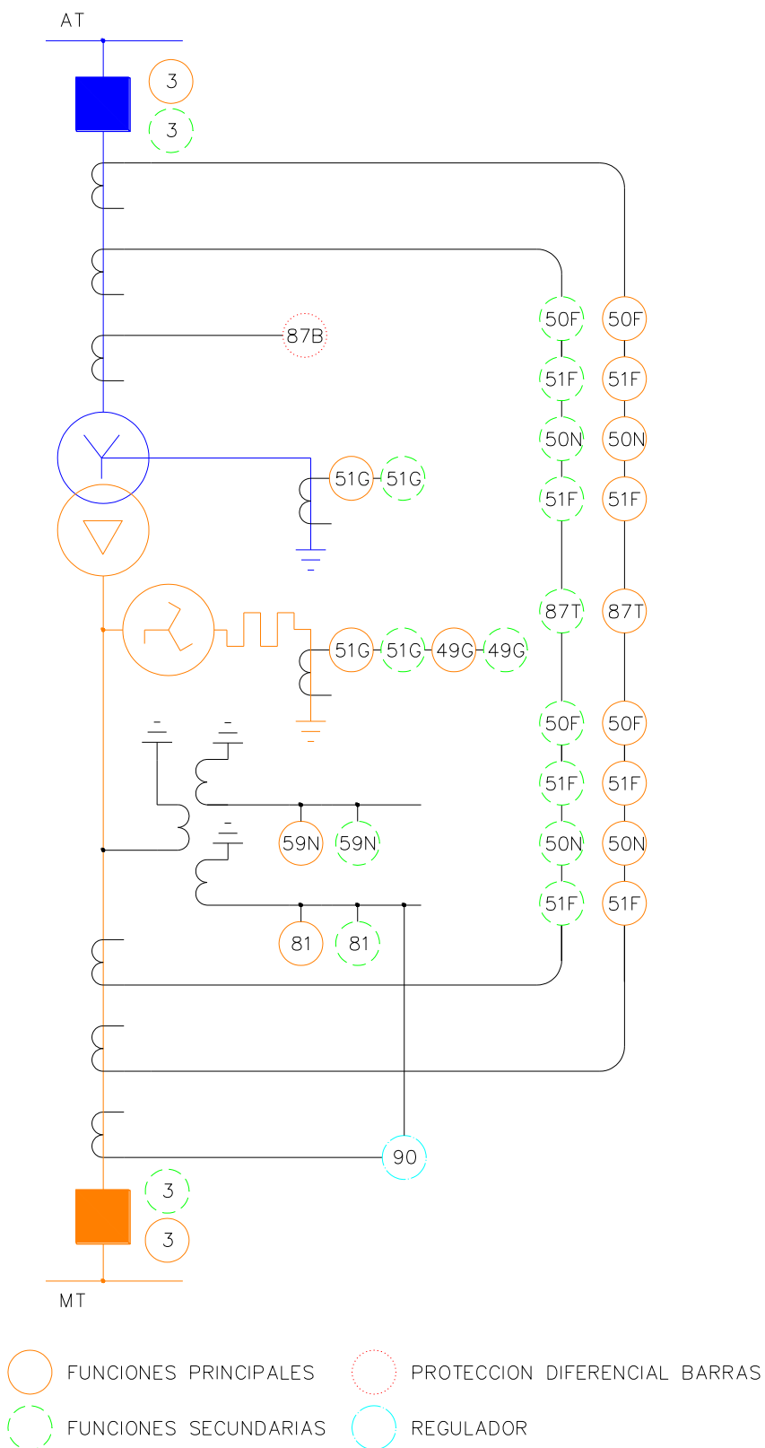
Figura 48.AT/MT
